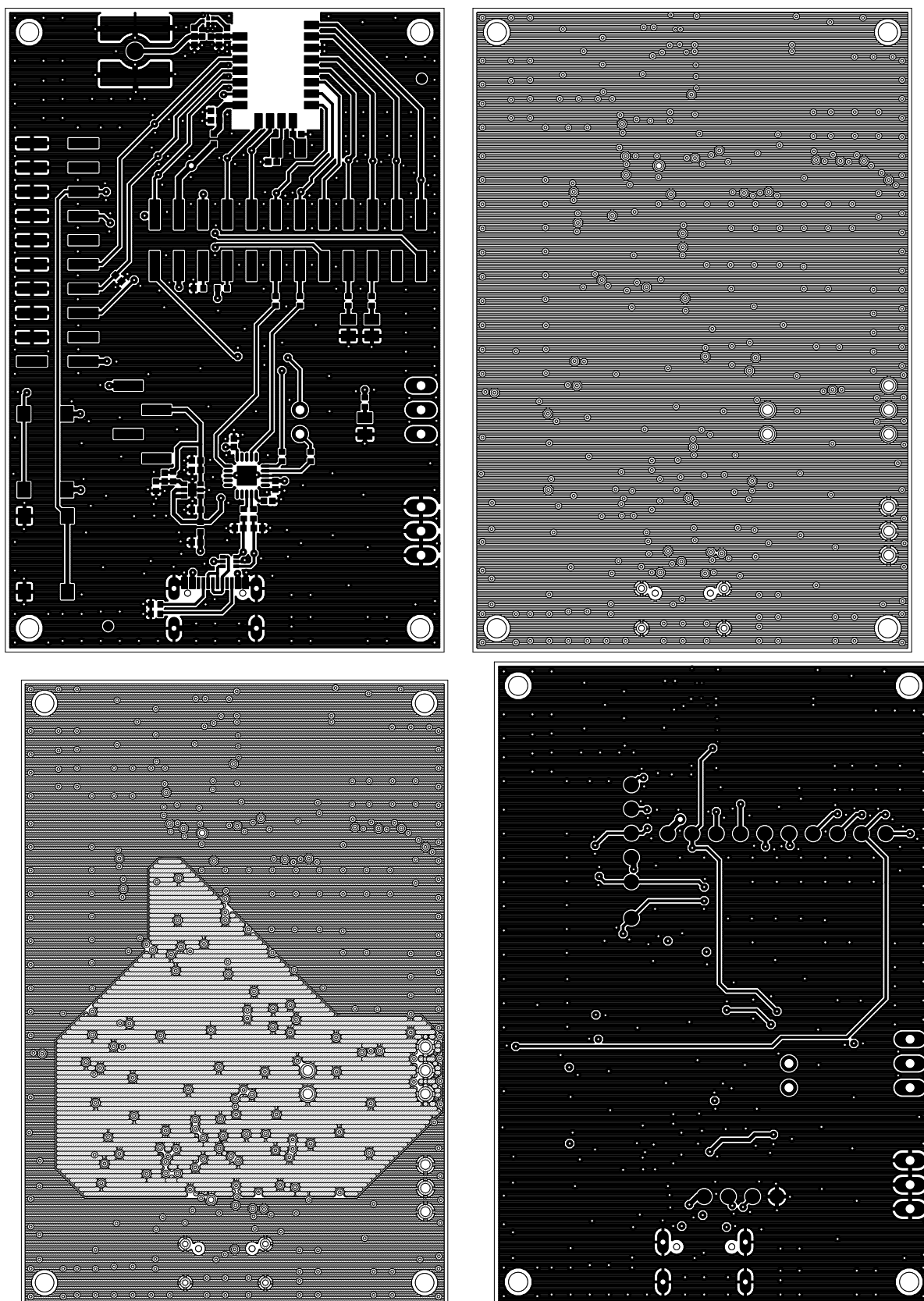
Figure 21: Top, Layer 2, Layer 3 and Bottom Layer
